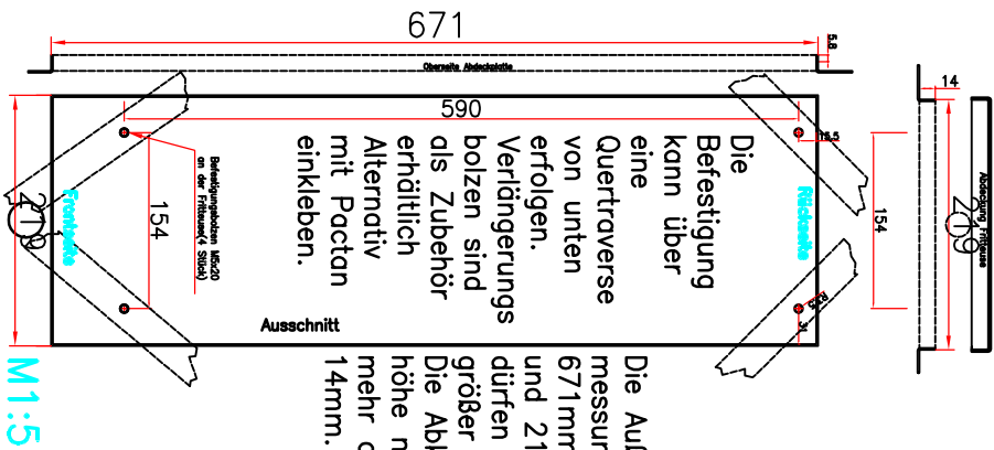
Einbauausschnitt für VXE 21
