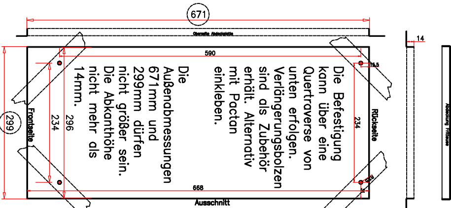
Einbauausschnitt für VXE 31
